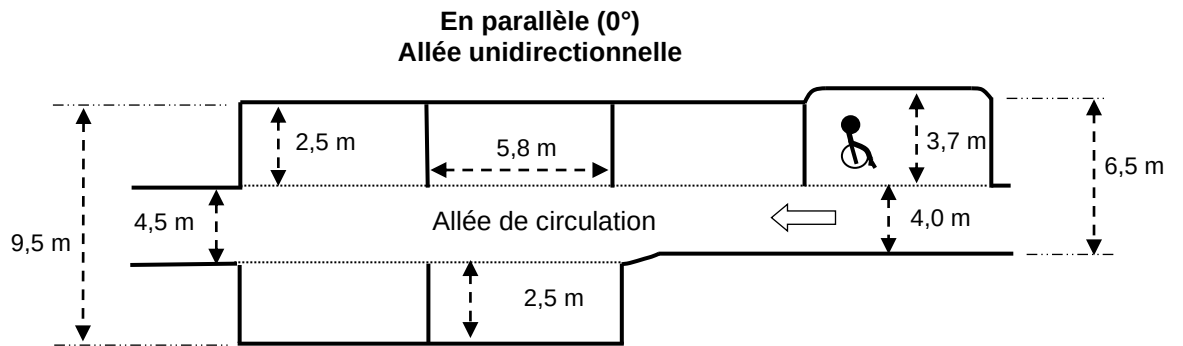
Illustration 10.11 Dimension des cases de stationnement et des allées de circulation
